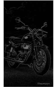
Prewitt Edge
